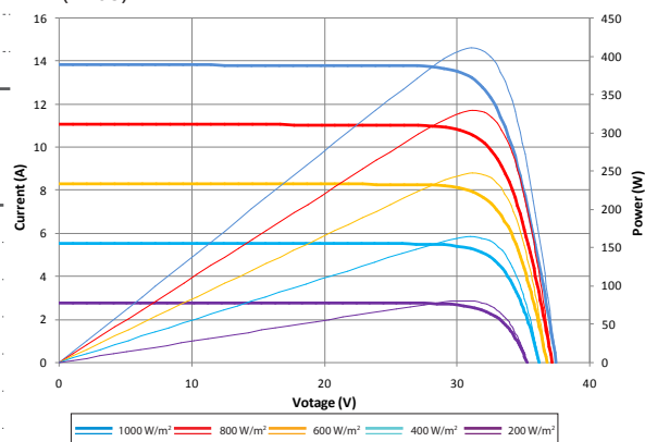
Wykres napięcia i mocy oraz napięcia i natężenia (410S)
