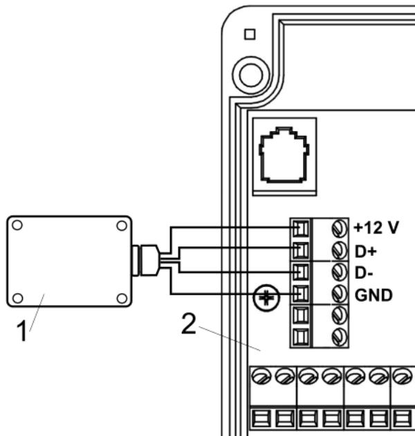
Podłączenie modułu do regulatora głównego ecoMAX850P2, R2, D2 : 1 - moduł radiowy, 2 - regulator główny.
