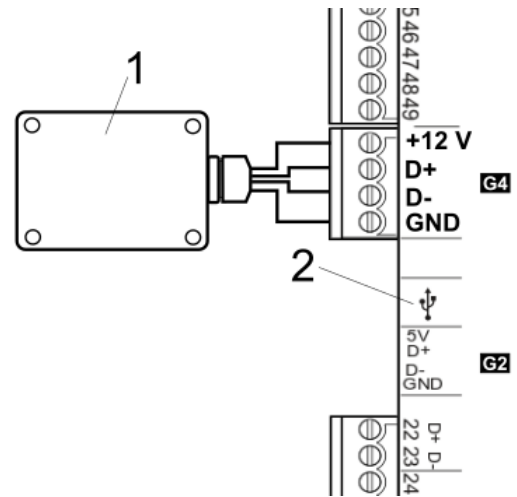
Podłączenie modułu do ecoMAX860P3, D3 : 1 - moduł radiowy, 2 - regulator główny.
