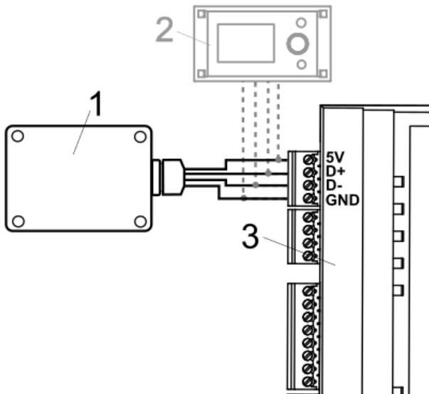
Podłączenie modułu do ecoMAX800P3, D3 oraz ecoMAXX800R3, T3 : 1 - moduł radiowy, 2 - panel sterujący, 3 - regulator główny.
