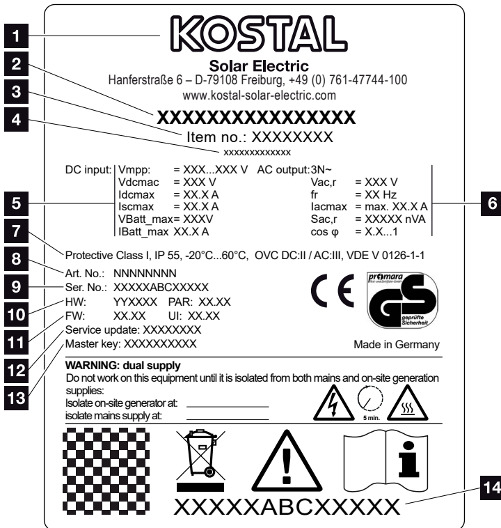
Ilustr. 77: Tabliczka znamionowa
