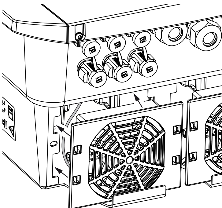
Ilustr. 75: Montaż wentylatora
