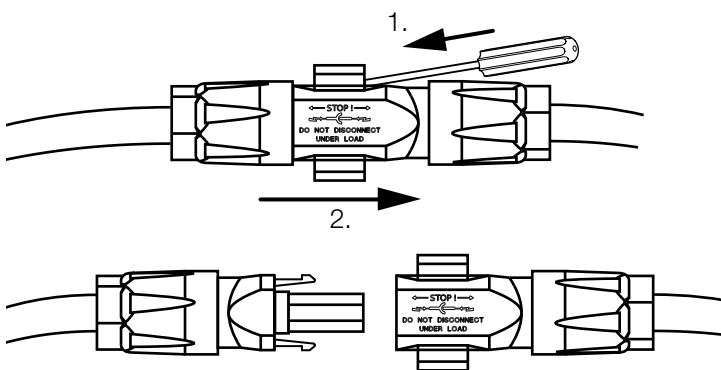
Ilustr. 41: Rozłączenie złącza DC SUNCLIX
