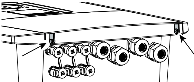
Ilustr. 21: Zdjęcie pokrywy
