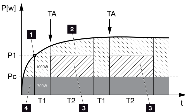
Ilustr. 66: Wykres dynamicznego zużycia własnego (funkcja 1)
