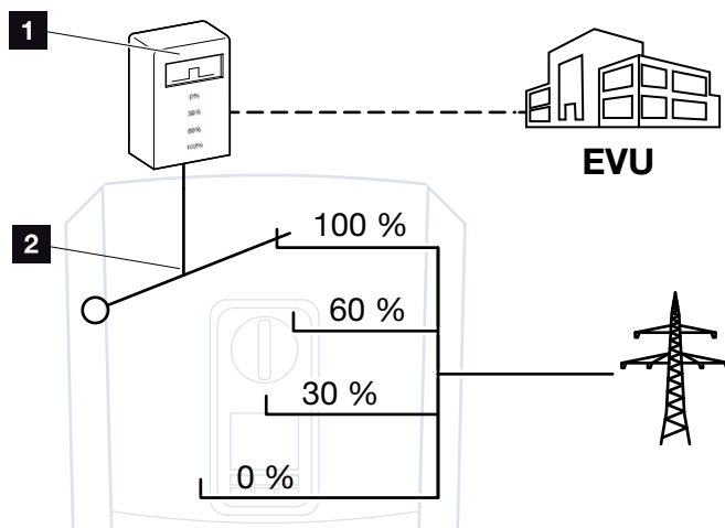
Ilustr. 59: Sterowanie mocą czynną za pomocą odbiornika do zdalnego sterowania
