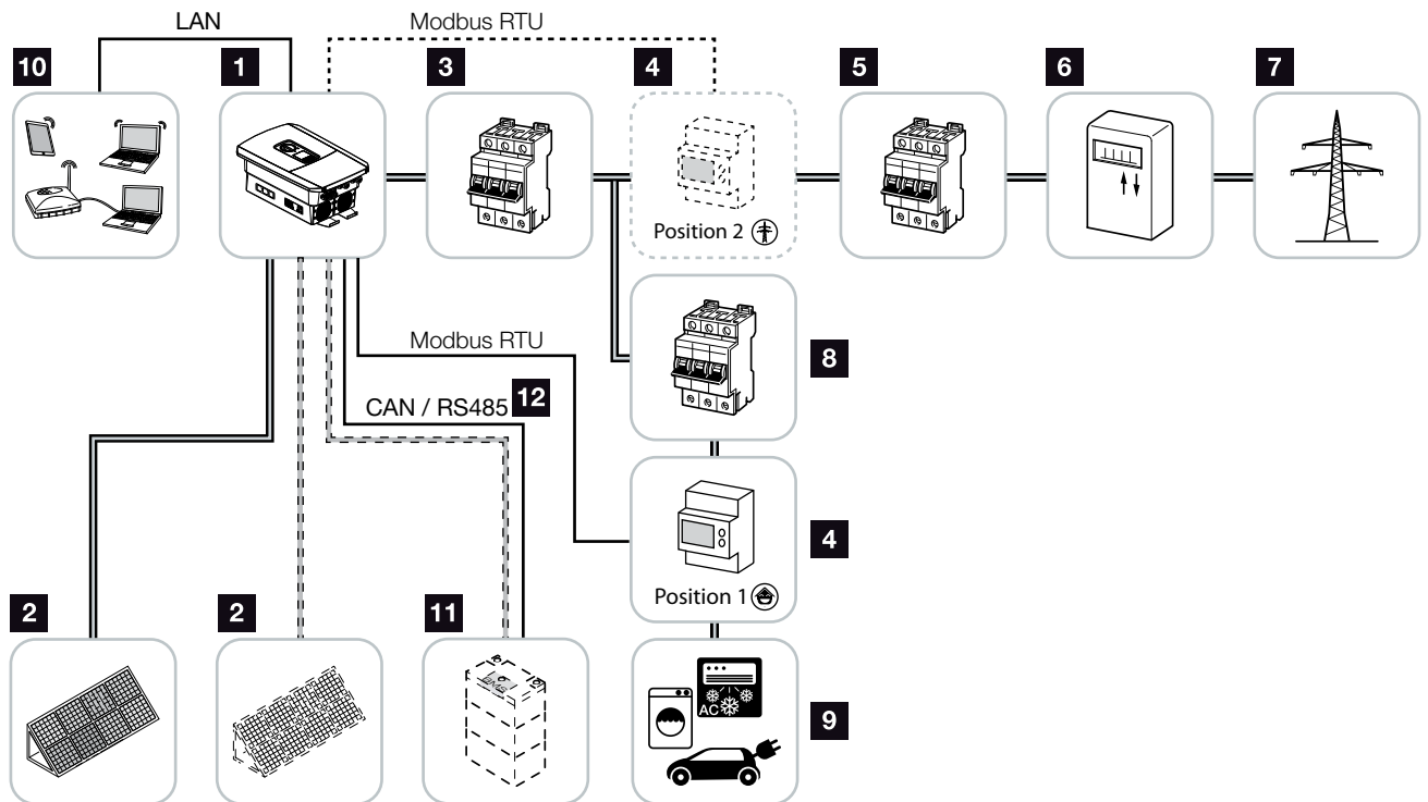
Ilustr. 8: Instalacja fotowoltaiczna z PV i złączem do akumulatora
