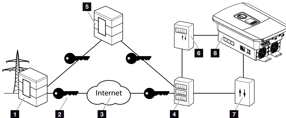
Ilustr. 61: Podłączenie inteligentnych systemów pomiarowych
