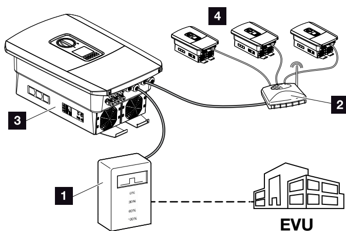
Ilustr. 60: Falownik z odbiornikiem do zdalnego sterowania
