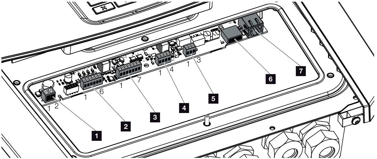
Ilustr. 26: Złącza Smart Communication Board
