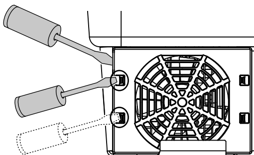
Ilustr. 72: Zwalnianie zatrzasków
