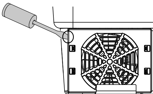
Ilustr. 71: Zwalnianie kratki wentylatora
