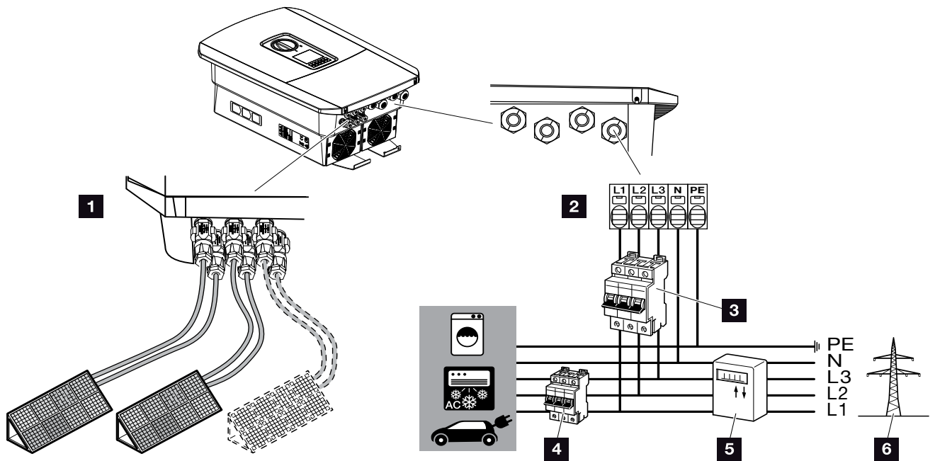
Ilustr. 20: Widok złączy elektrycznych
