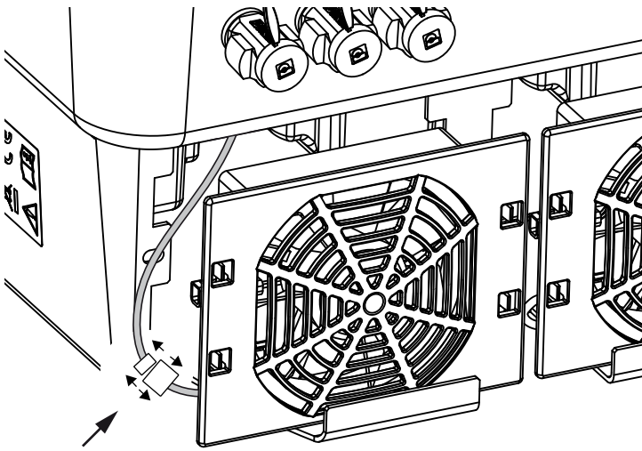
Ilustr. 73: Odłączenie kabla wentylatora
