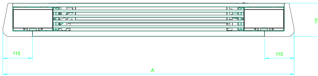
SLS wersja niska - przyłącza bez armatury przyłączeniowej
