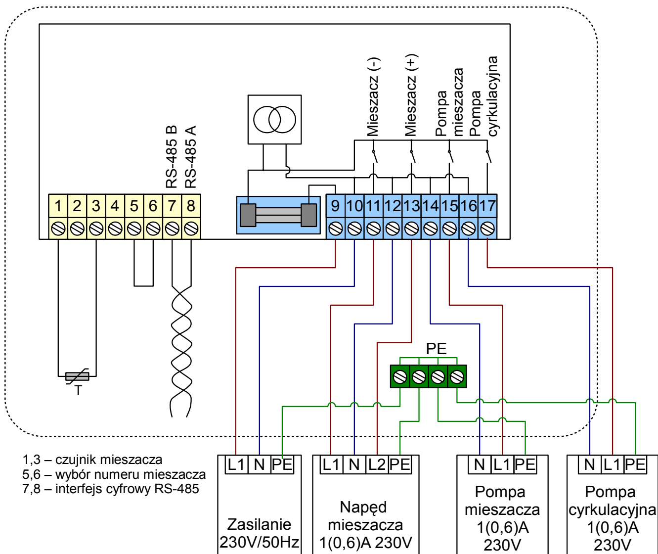
Rysunek 3: Podłączenie modułu R803BB
